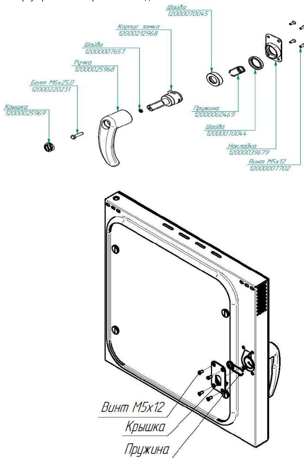
Рис.6. Ремонт замкового устройства
